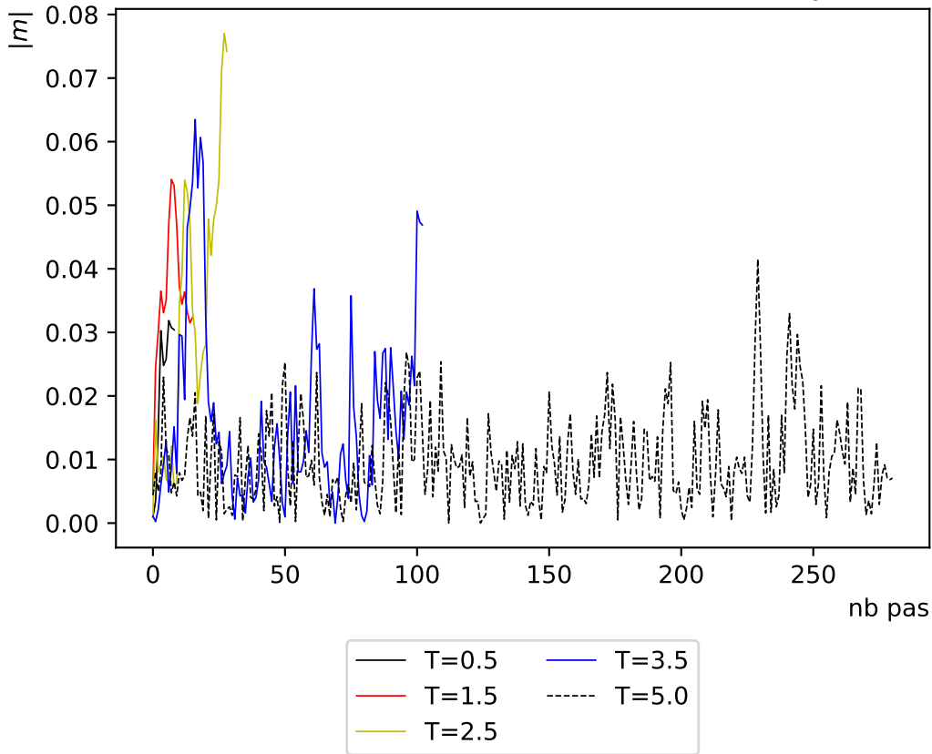
Evolution de l'aimantation sur critère \pm 5\% de la moyenne, N=128
